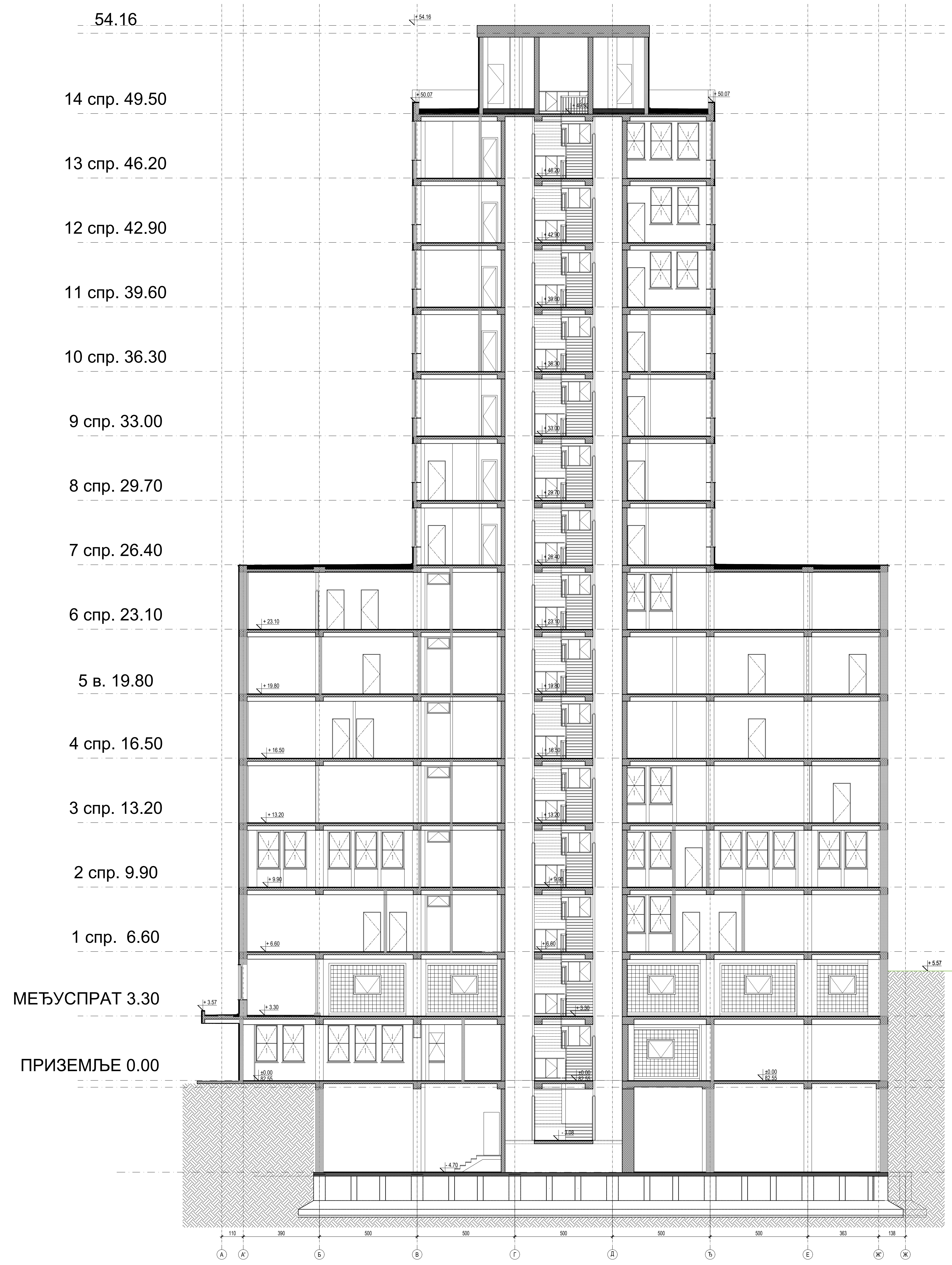
ПРЕСЕК 2-2
