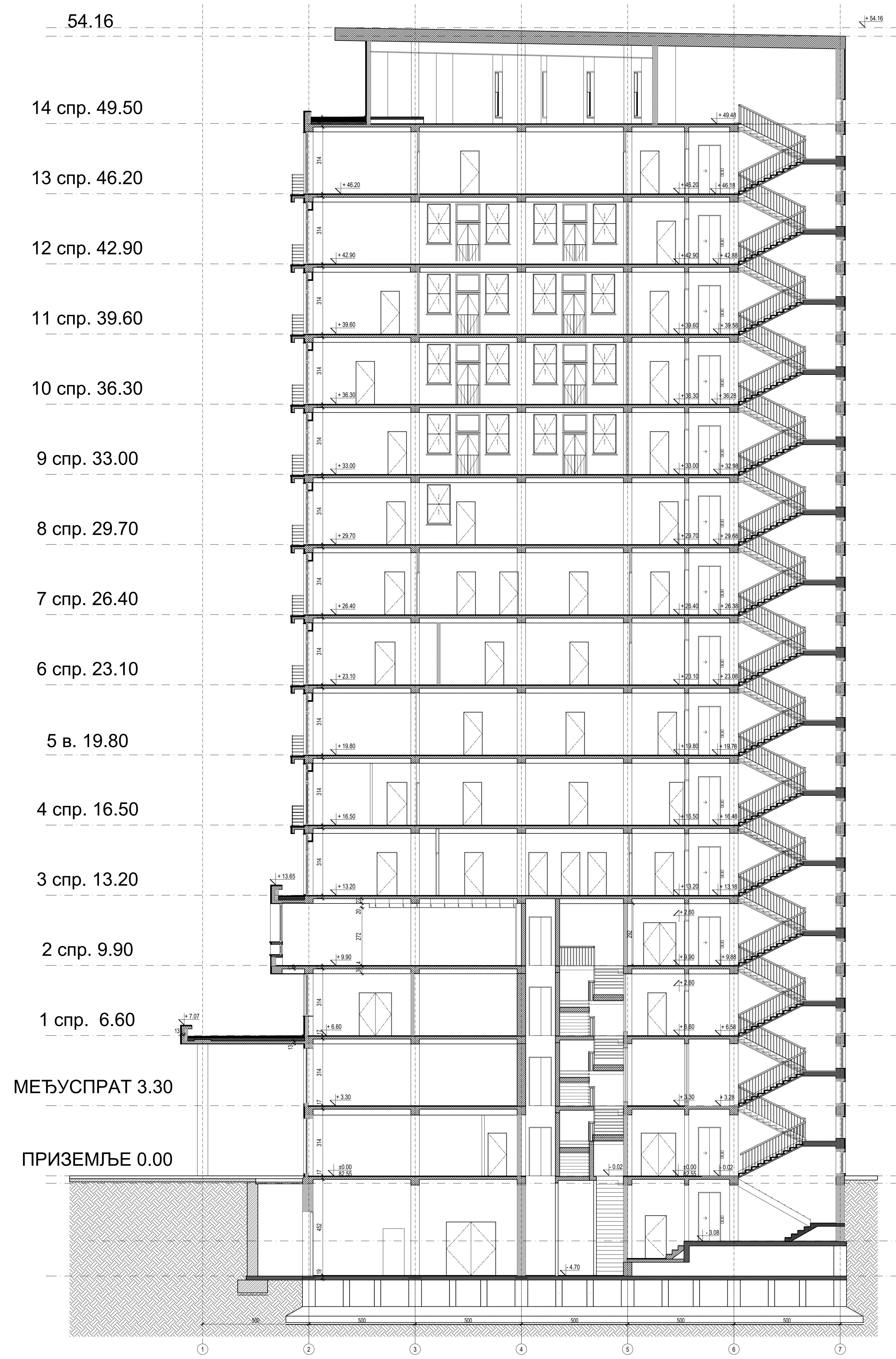
ПРЕСЕК 1-1
